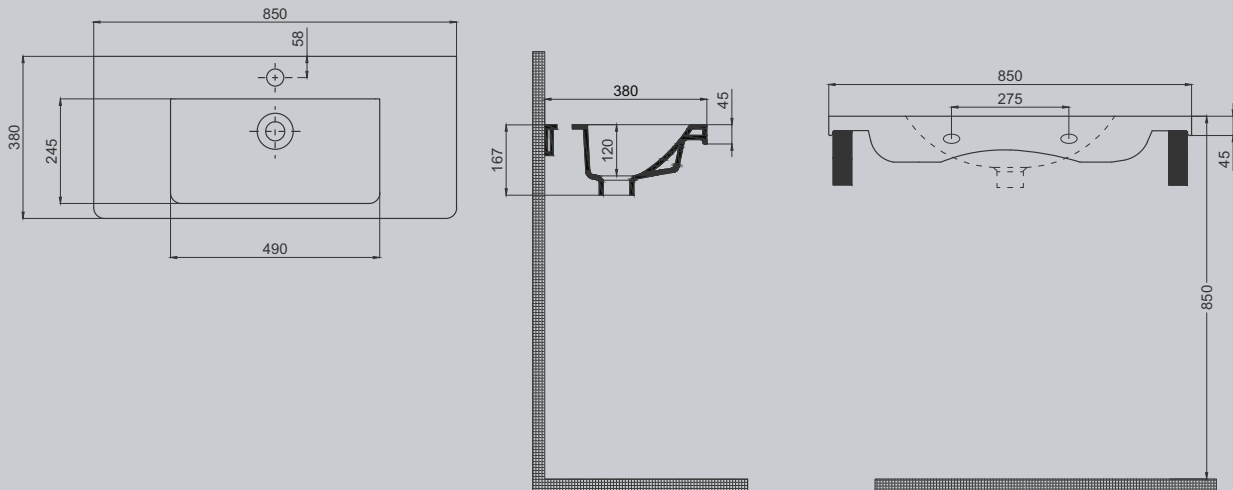
Space Line-S Mobilya Uyumlu Lavabo |70SP21085.00.1.3.01
