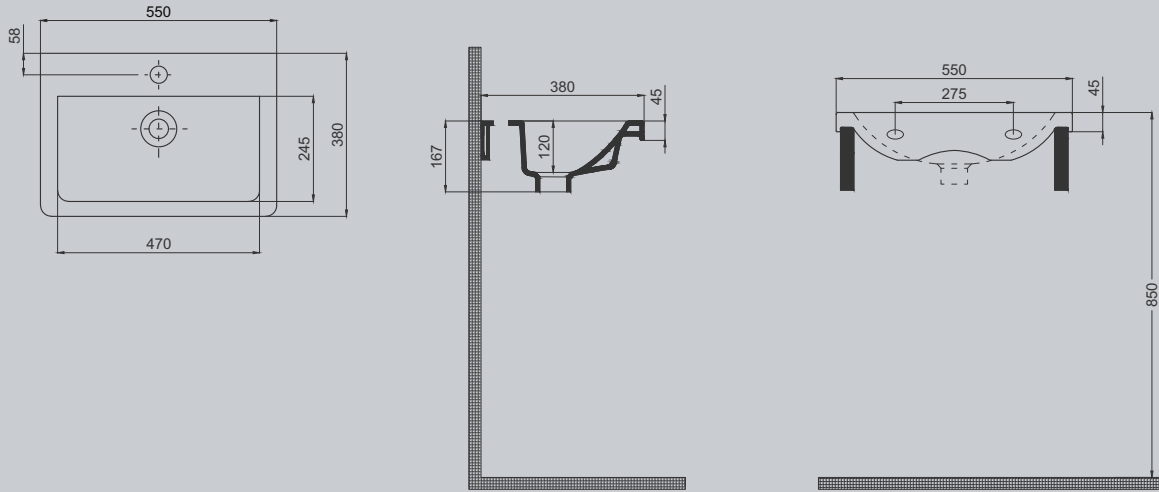
Space Line-S Mobilya Uyumlu Lavabo |70SP21165.00.1.3.01
