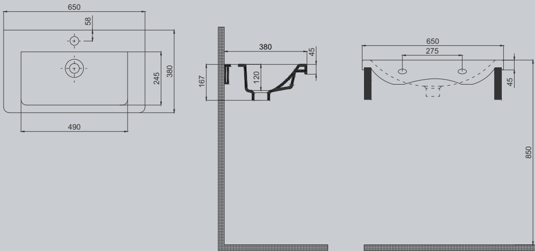
Space Line-S Mobilya Uyumlu Lavabo |70SP21085.00.1.3.01
